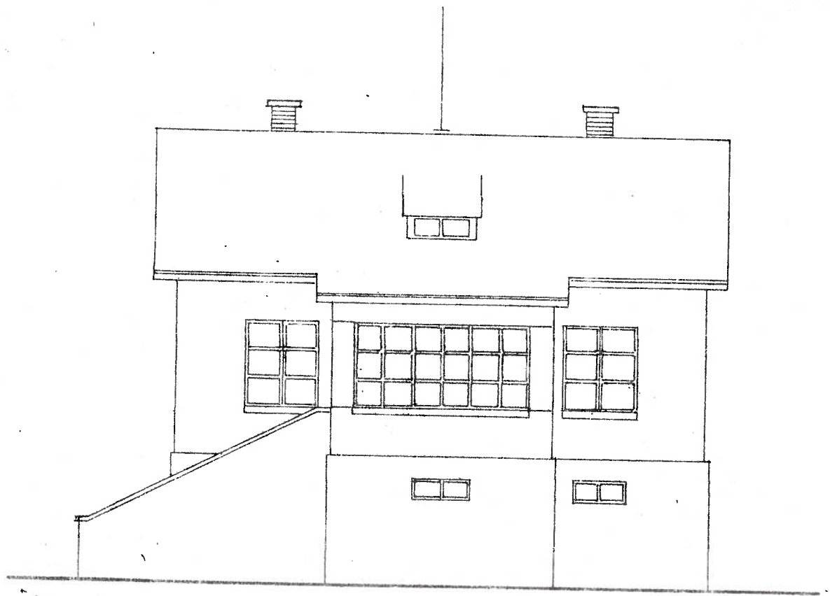
POHLED JÍŽNÍ
