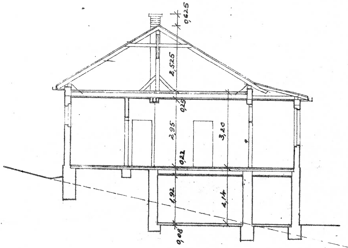
REZ A-B
